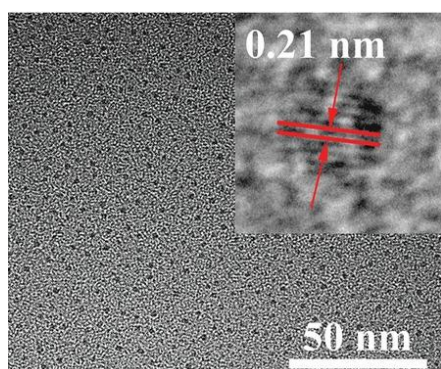
Рис. 2. TEM и HRTEM (во врезке) изображение “красных” углеродных точек.
