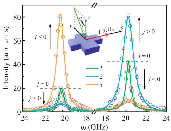
Рис. 1. В центре: исследуемая гетероструктура “крест Холла”, намагниченная в плоскости. Внешнее магнитное поле H и поле обменного смещения H_{ex} направлены параллельно друг другу в плоскости пленки. Свет падает в плоскости, перпендикулярной магнитным полям. Спектры рассеяния Манделштама-Бриллюэна при нулевом токе (зеленая кривая 1), при токе вдоль магнитного поля (синяя кривая 2) и в противоположном направлении (оранжевая кривая 3). По горизонтальной оси разность частот: частоты исходного лазерного излучения (532 нм) и частоты рассеянного света. Стоксова компонента оказывается справа, антистоксова – слева.
