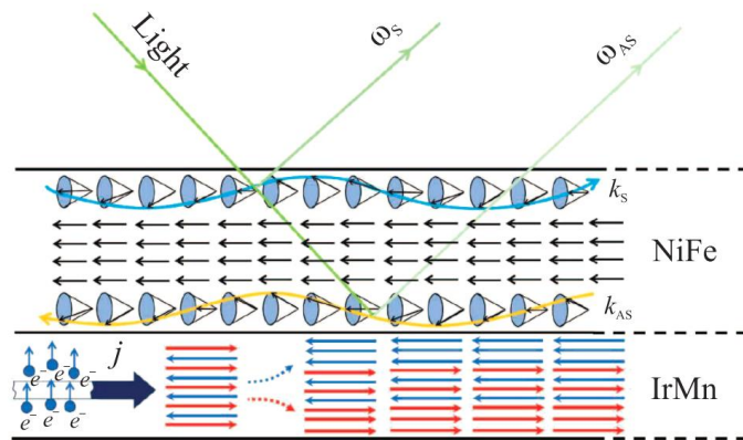
Рис. 2. К механизму влияния тока на рассеяние Манделштама-Бриллюэна.
